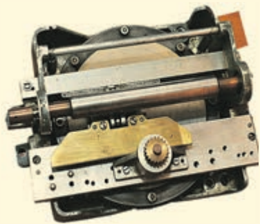
Грибовидный фрикционный интегратор.
