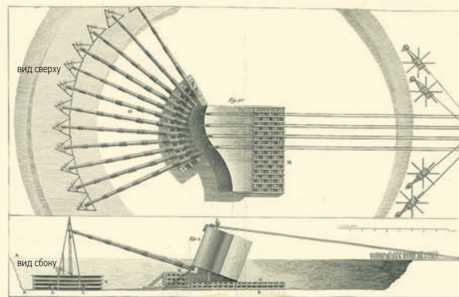
Перемещение валуна с помощью лебедок
